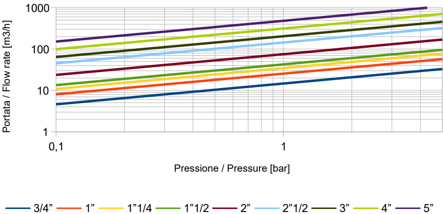
Filtro Acqua - Water Strainer Art. 0006 / 2006 / 7006 / 0106 / 2106 / 7106 "VENEZIA"
