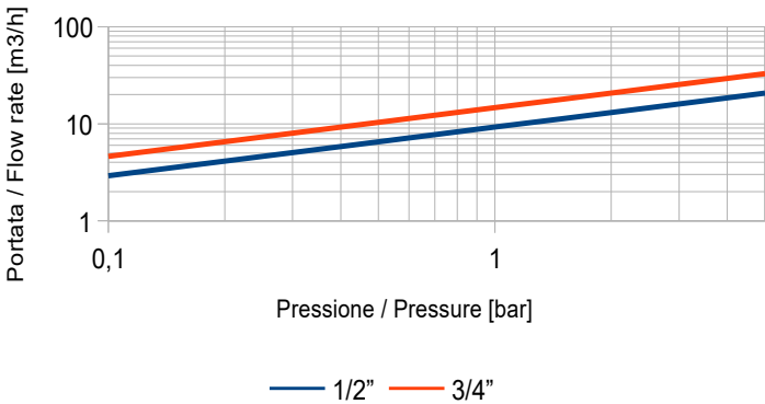
Filtro Acqua - Water Strainer Art. 0007 / 0107 / 7007 / 7107 "PISA"
