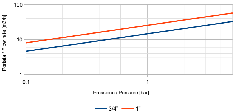
Filtro Acqua - Water Strainer Art. 2007 "PISA"
